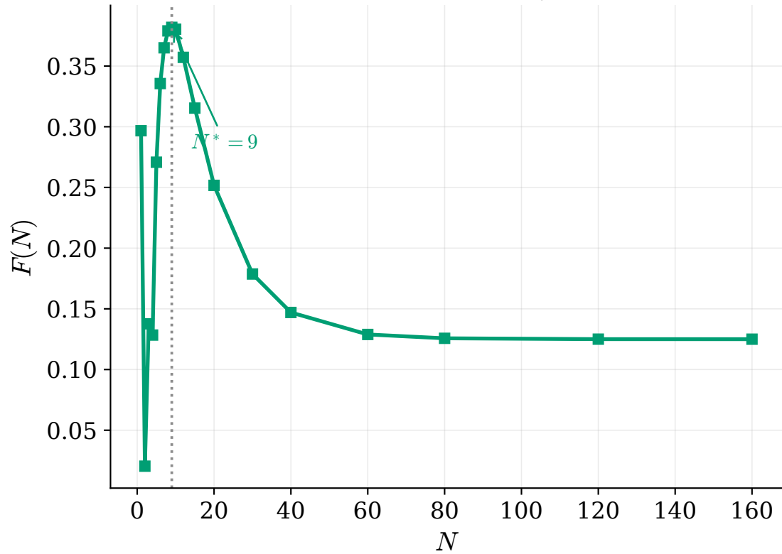
Scenario B ( R_0 , da |000\rangle )
