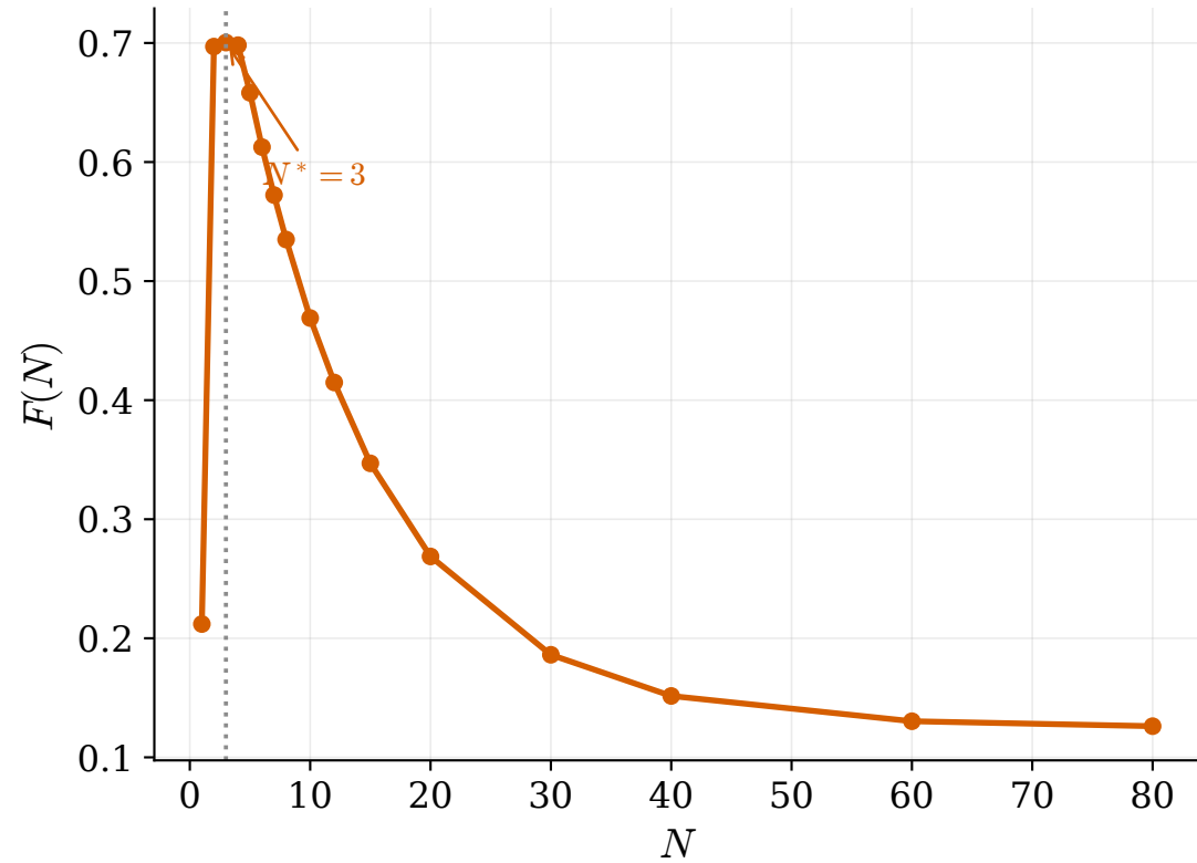
Scenario A (preparazione VQE)
